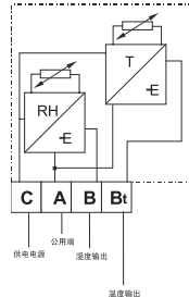
0 ... 10 V 输出接线图
