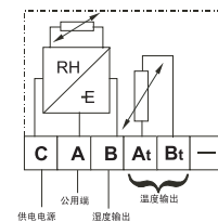
带 NTC K2, A99, Pt1000 温度输出接线图
