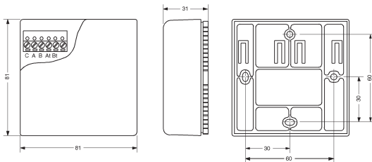
室内型传感器 HT-90xx-URW 尺寸 (mm)
