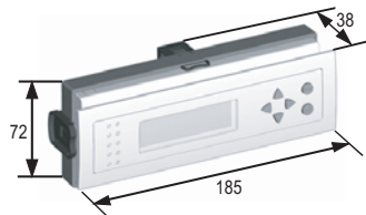
面板安装型尺寸(mm)
