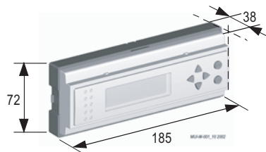
墙面安装型尺寸(mm)
