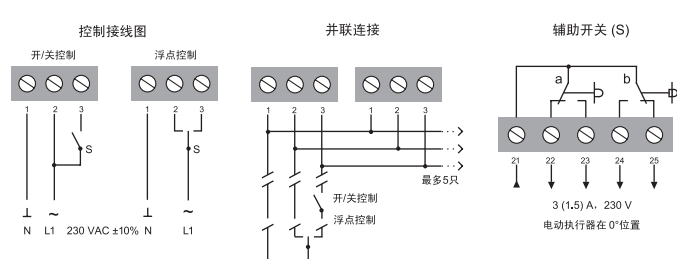
M9108 ADx 1接线图
