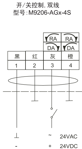
M9206-AGx-4S接线图
