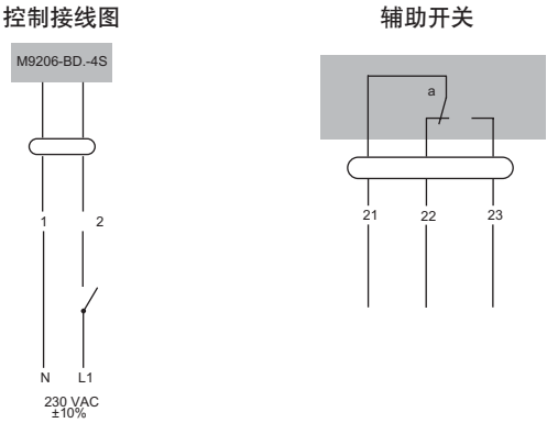
M9206-BDx-4S接线图
