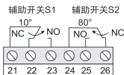
辅助开关 型号: M9216-AGC-2
