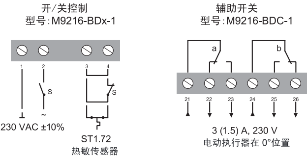
M9216-BDx-1接线图
