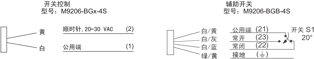
M9206-BGx-4S接线图
