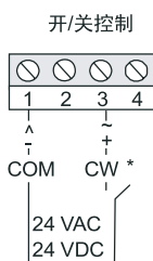
M9216-AGx-2接线图
