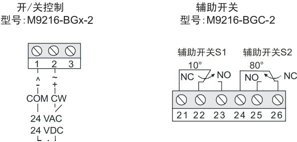
M9216-BGx-2接线图
